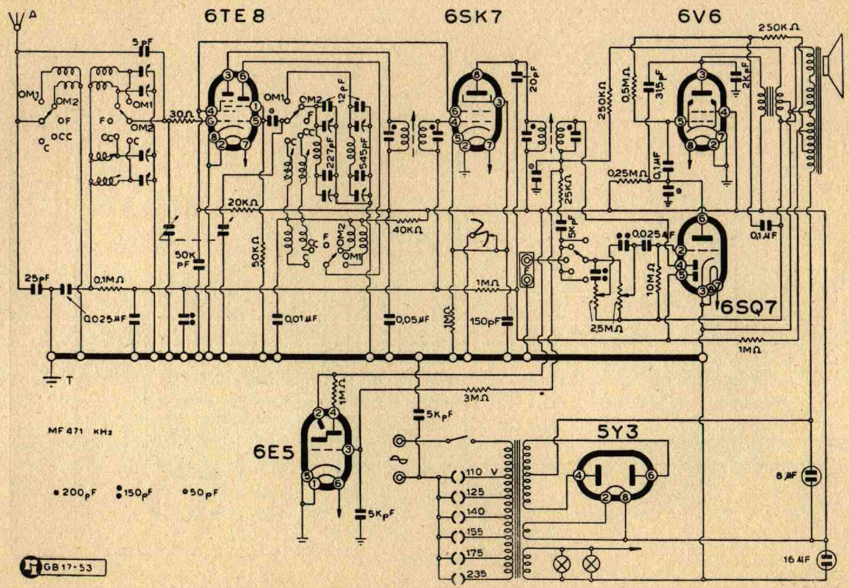
Lo schema elettrico dell' SV 62
